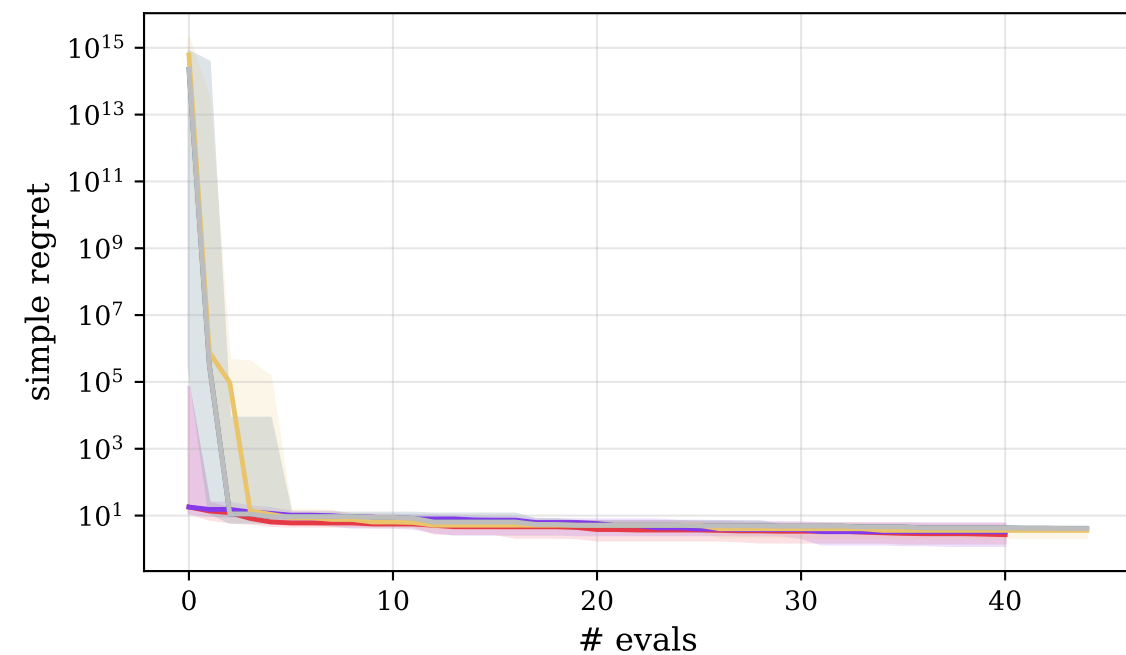
TensionSpring
